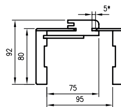
Schnitt ORB 075
