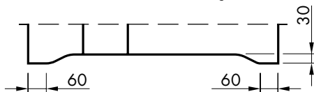
Unterschnitt in Vetro D Türflügeln
