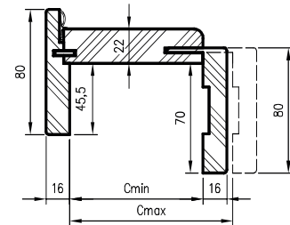
Querschnitt des Türrahmens
