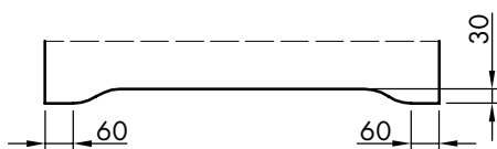
Standard-Unterschnitt in Türflügeln
