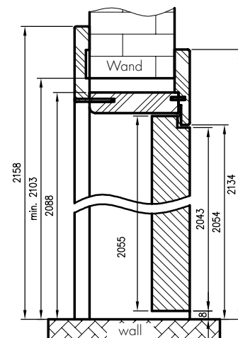
Vertikalschnitt ORO
