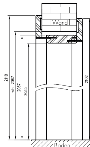
Vertikalschnitt des verstellbaren Tunnels mit Winkel. T63
