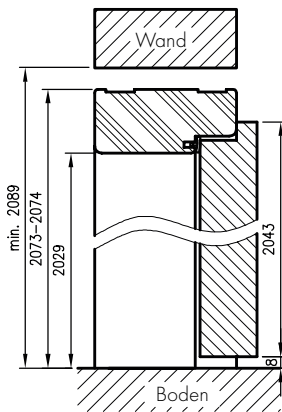
VERTIKALSCHNITT OP FÜR TÜRFÜGEL MIT FALZ
