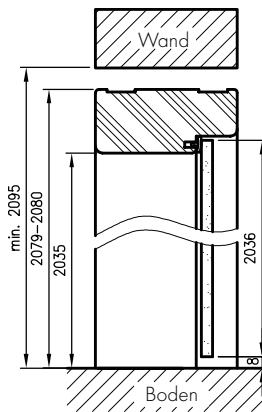
VERTIKALSCHNITT OP FÜR GLASTÜRFÜGEL
