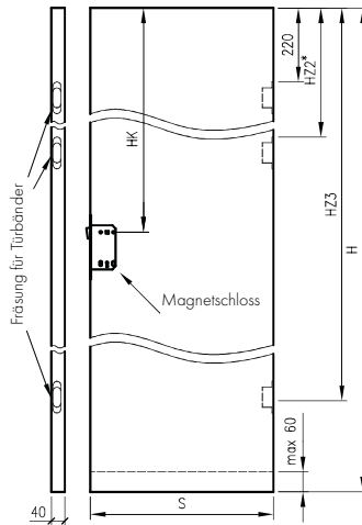
Türflügel ohne Falz: Standard 10, Modern, Plus
