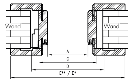
Horizontalschnitt OR/ORC
