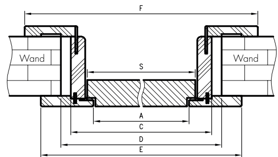
Horizontalschnitt ORO
