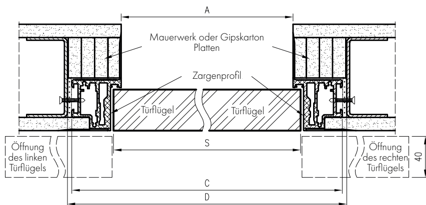
Querschnitt Sara Eco 2 Tür ohne Falz nach außen öffnend
