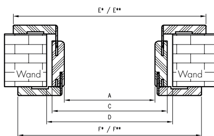
Querschnitt TUN
