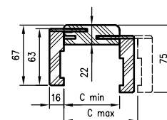
Schnitt TUN-Profil mit Winkel. T63
