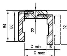
Schnitt TUN-Profil mit Winkel. T80
