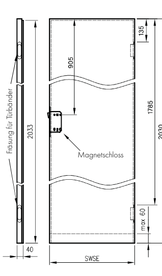
Türflügel ohne Falz Sara Eco 2 im Standard 202X
