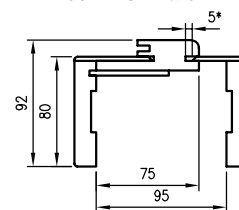
Schnitt ORB 075
