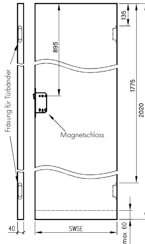
A - Führungsfräsung
