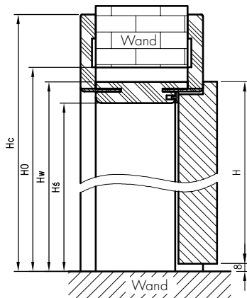
Vertikalschnitt OR
