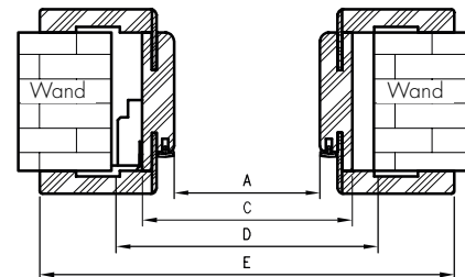
Horizontalschnitt OR
