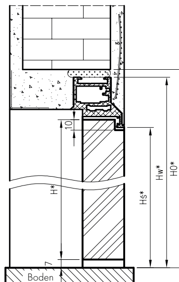
Vertikalschnitt Sara Eco 2 Tür mit Falz nach außen öffnend
