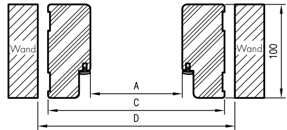
HORIZONTALSCHNITT OP
