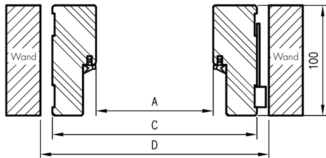
Horizontalschnitt OPB
