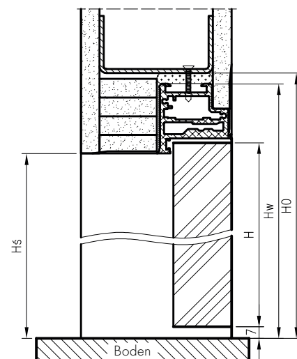
Vertikalschnitt Sara Eco 2 Tür ohne Falz nach außen öffnend
