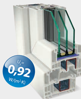
Schmalen Rahmen mit Flügel und bestätigter ift-Passivhaustauglichkeit
